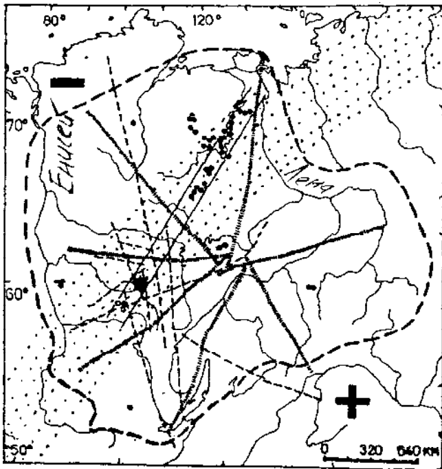
Рис. 1. Крупные тектонические зоны в районе Тунгусского события (по данным Г.Г.Кочемасова)
